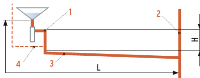
Figura 14.2 – conductă de legătură ventilată
