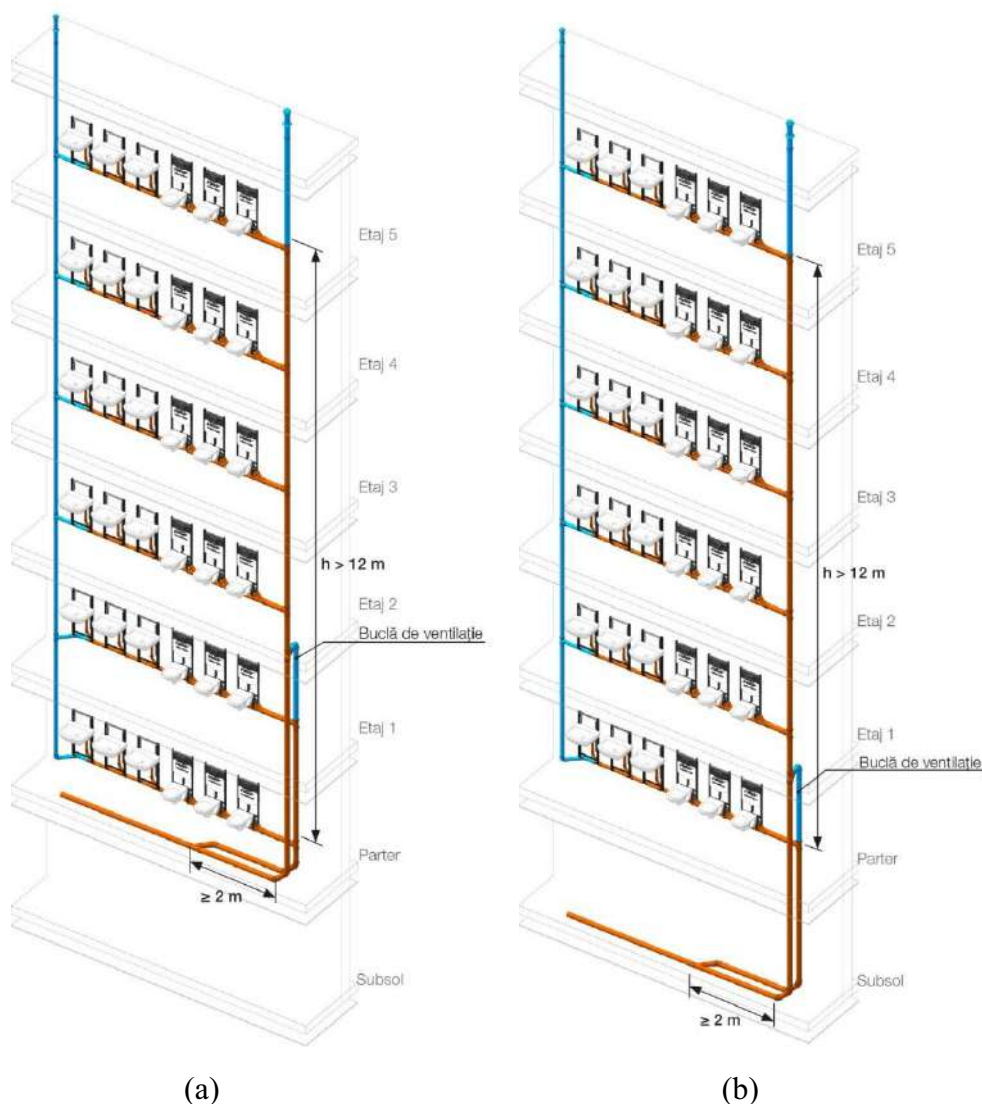
Figura A 5.9.11 (a), (b) – Variante suplimentare de ventilare secundară, pentru clădiri cu peste 5 niveluri, pentru care h > 12\text{ m} . Dotarea cu ventilare secundară se realizează în condițiile descrise în capitolul 13.
