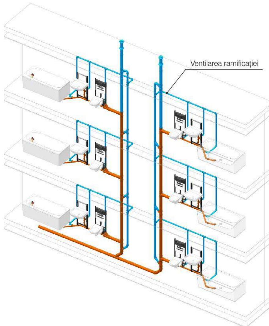
Figura A5.9.7 – Exemple de ventilară primară, secundară și auxiliară, aplicate unei instalații de canalizare pentru o clădire cu maxim 3 niveluri; dotarea cu ventilară secundară și auxiliară se realizează în condițiile descrise în capitolul 13.
